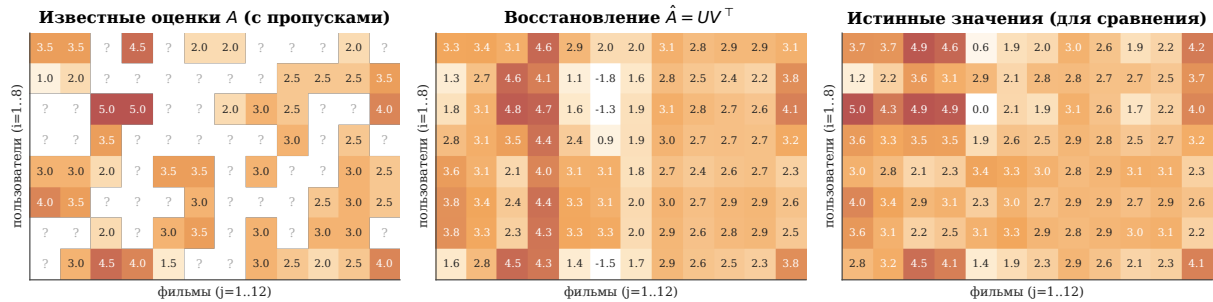
Рис. 4.22. Иллюстрация задачи Netflix на маленьком примере: 8 пользователей, 12 фильмов, ранг r = 2 . Слева — известные оценки (большинство клеток помечены '?'). В центре — восстановление \hat{A} = UV^T с r -факторизацией (все клетки теперь заполнены, в том числе неизвестные). Справа — истинные значения (для проверки). Метод не просто заполняет пропуски, но и обнаруживает скрытые (латентные) закономерности в данных.
