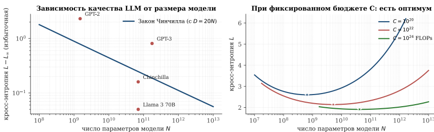
Законы скейлинга Чинчилла: L(N, D) = L_{\infty} + A/N^{0,34} + B/D^{0,28}
